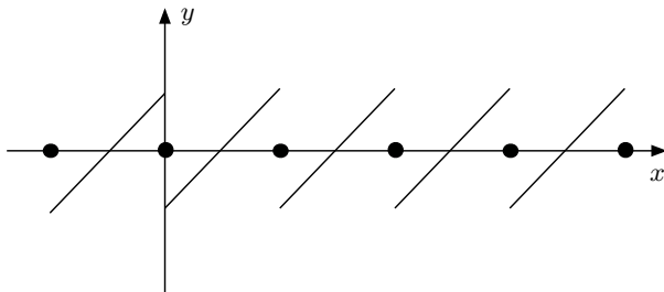
Fig. 7.1. The sawtooth function y = ((x)) .
